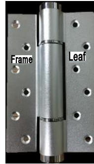
Empty Hinge
